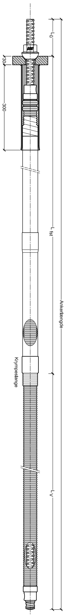
Med vinkeludligningsrør. Følgende dele korrosjonsbeskyttes iht. DIN EN ISO 12944-5
