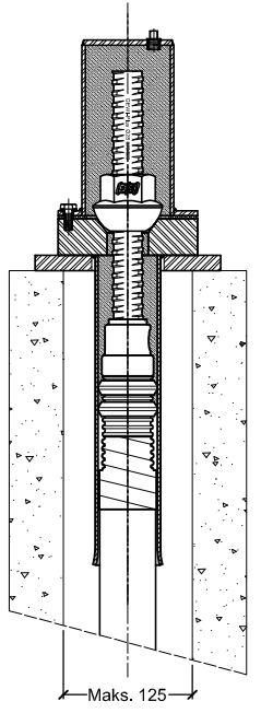
Over større borehul - skal efterfølgende udstøbes
